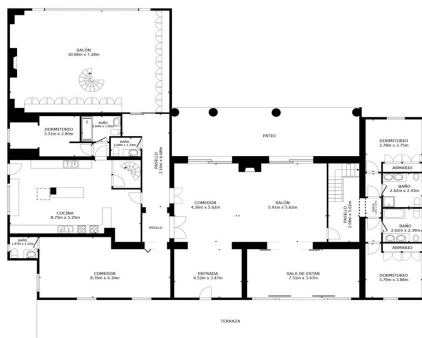
PLANTA 2
